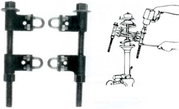
Compresseur de ressort d'amortisseur.
